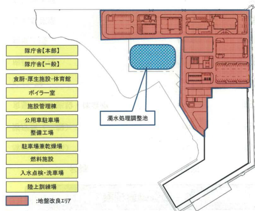
崎辺分屯地（仮称）全般配置図
